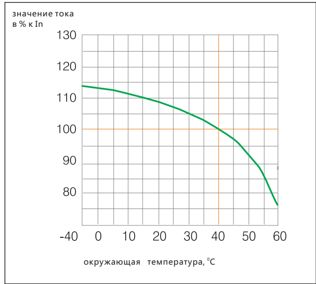
Характеристика температурной зависимости выключателя NM1-400
