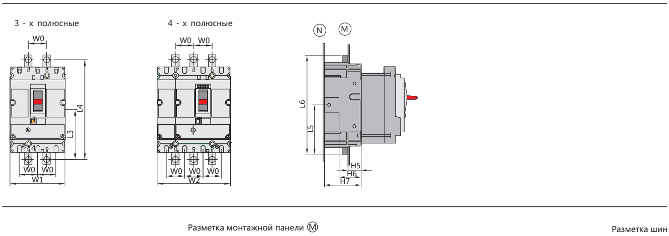
Расположение монтажных панелей
