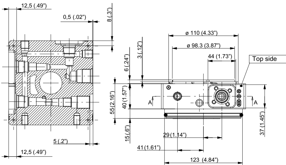
Sec. A-A
